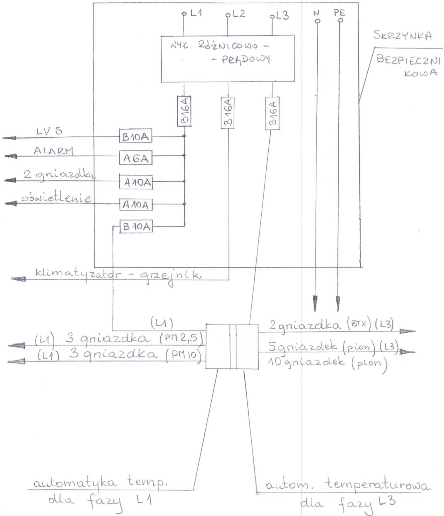
Rys. nr 5a - schemat zabezpieczeń, połączeń, obciążeń faz
