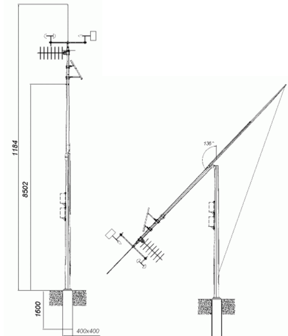
Rysunek 2a Maszt meteorologiczny
